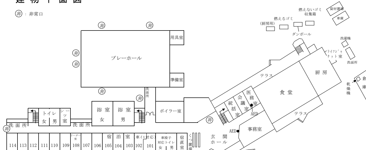
1 階 平 面 図
